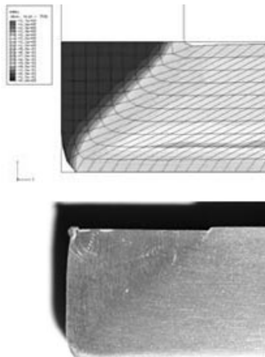
Figura 1: a) Simulación por elementos finitos de ECAE. b) Fotografía de una muestra procesada por ECAE.
