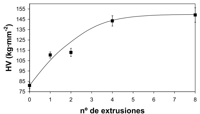
Figura 5: Dependencia de la dureza con el número de extrusiones ECAE
