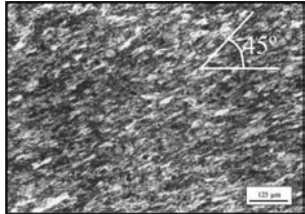
Figura 4: Micrografía de la microestructura obtenida tras una extrusión ( \gamma=2 , \epsilon \sim 1,2 ) en la sección longitudinal.
