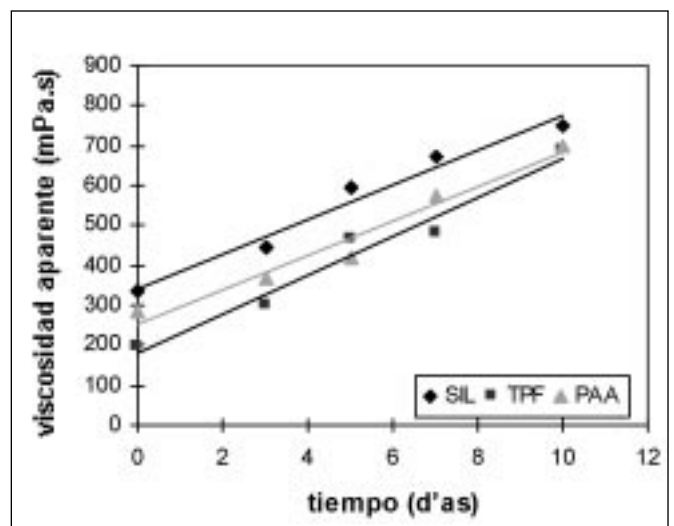
Fig. 4. Curvas de viscosidad aparente (a 200s -1 ) (cP) vs. tiempo de almacenamiento (días) para suspensiones de esmalte al 65% de sólidos, preparadas con 95 % fritas, 5% caolín, 0,5% CMC MV y distintos defloculantes a la concentración óptima.
